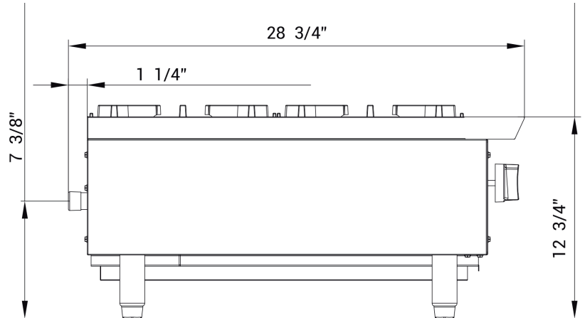
Vista Lateral
