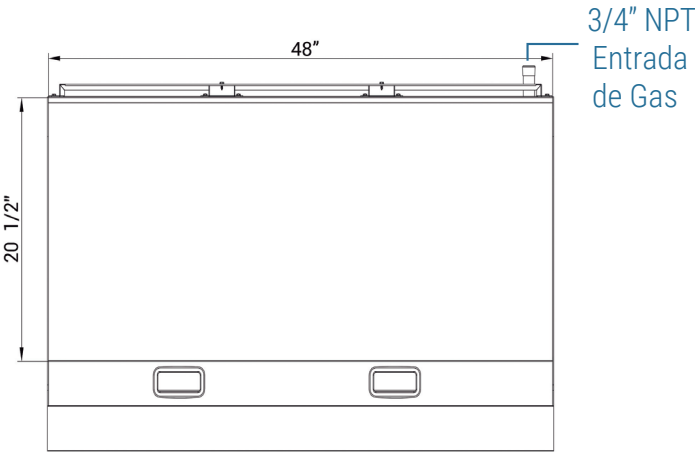
Vista Superior
