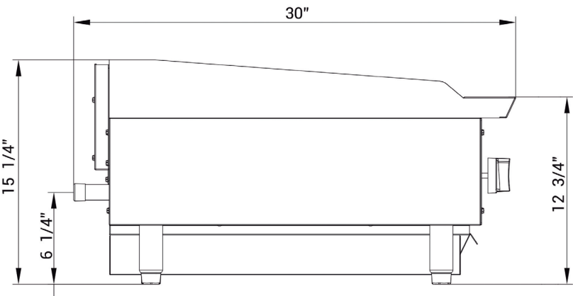
Vista Lateral
