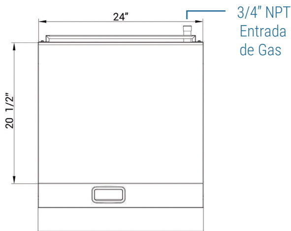
Vista Superior
